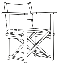
METTEUR-EN-SCÈNE F104 L58 P60 H84
